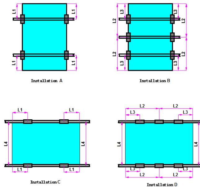
Fig 3: Parameters of double glass PV module
